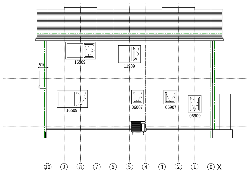
北 立面図
