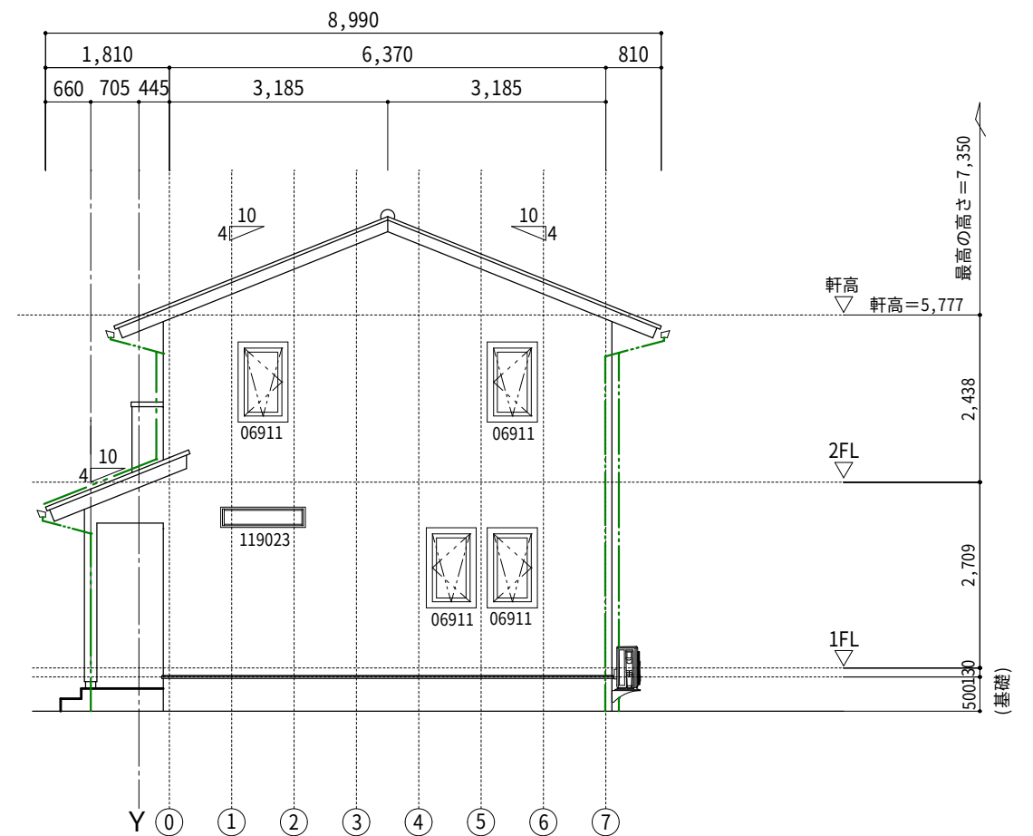
東 立面図
