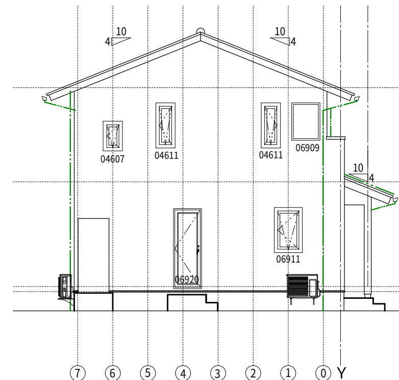
西 立面図
