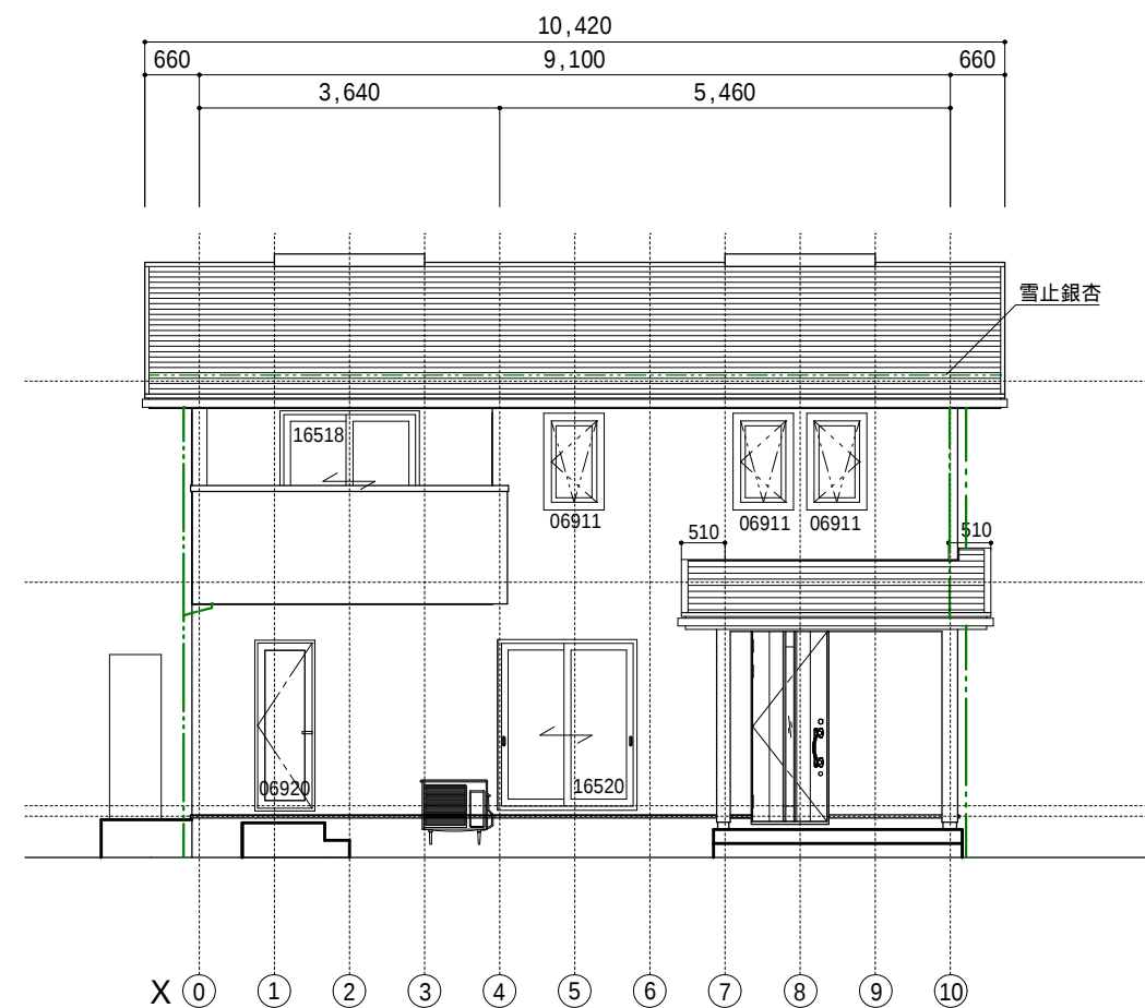
南 立面図
