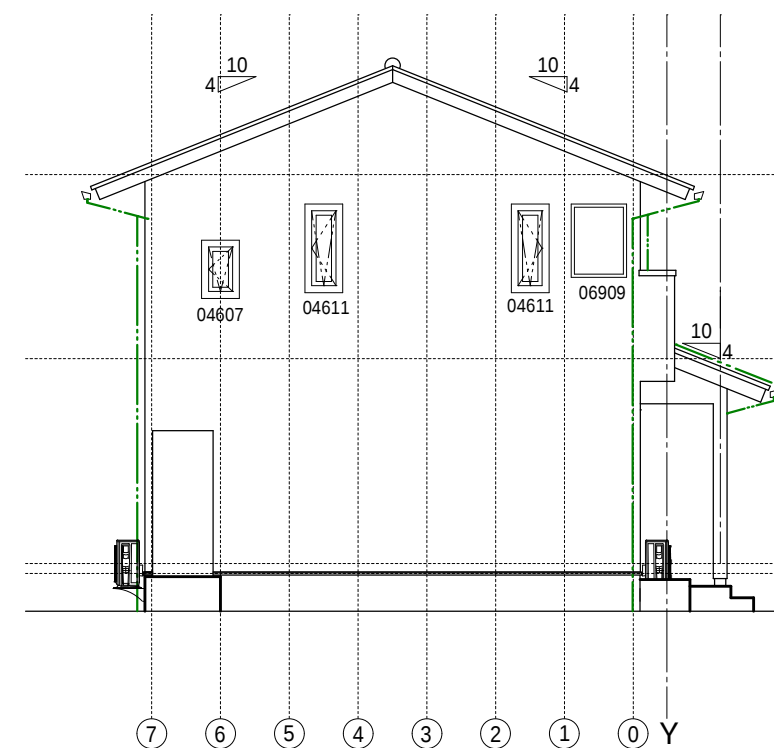
東 立面図
