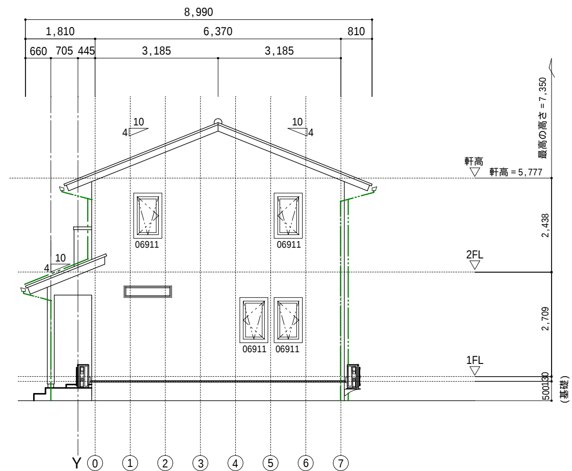
東 立面図
