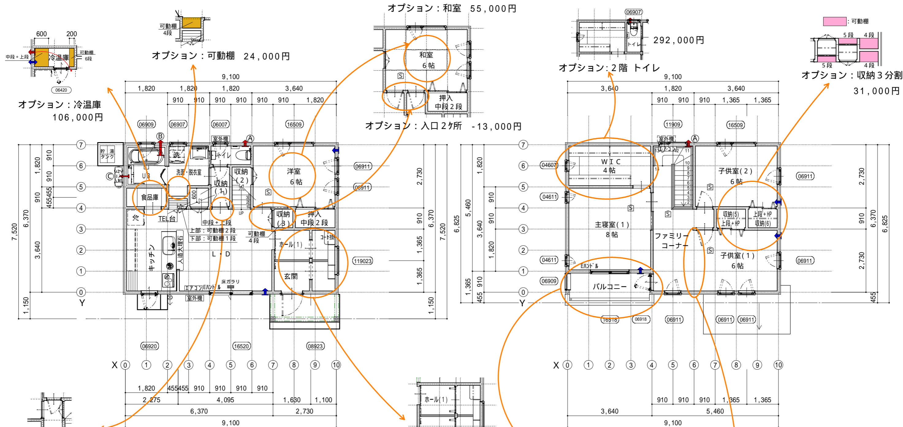
1階 平面図
