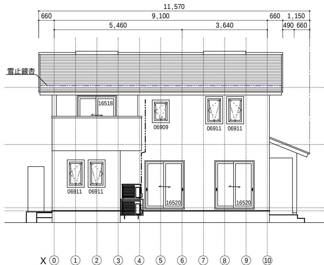
南 立面図
