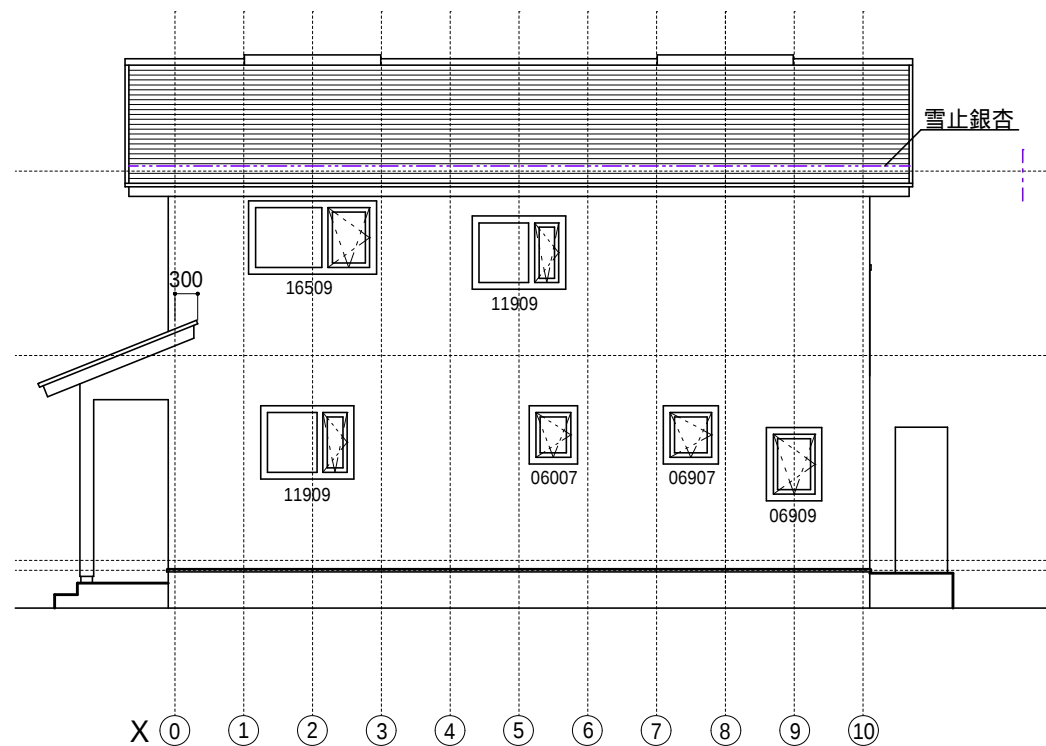
北 立面図
