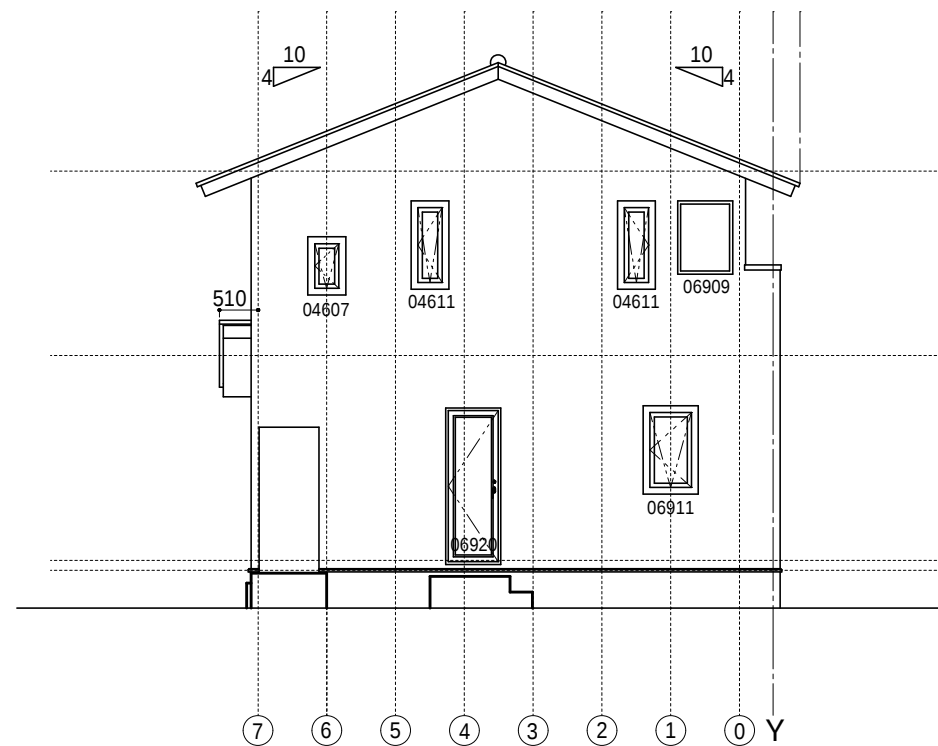
西 立面図
