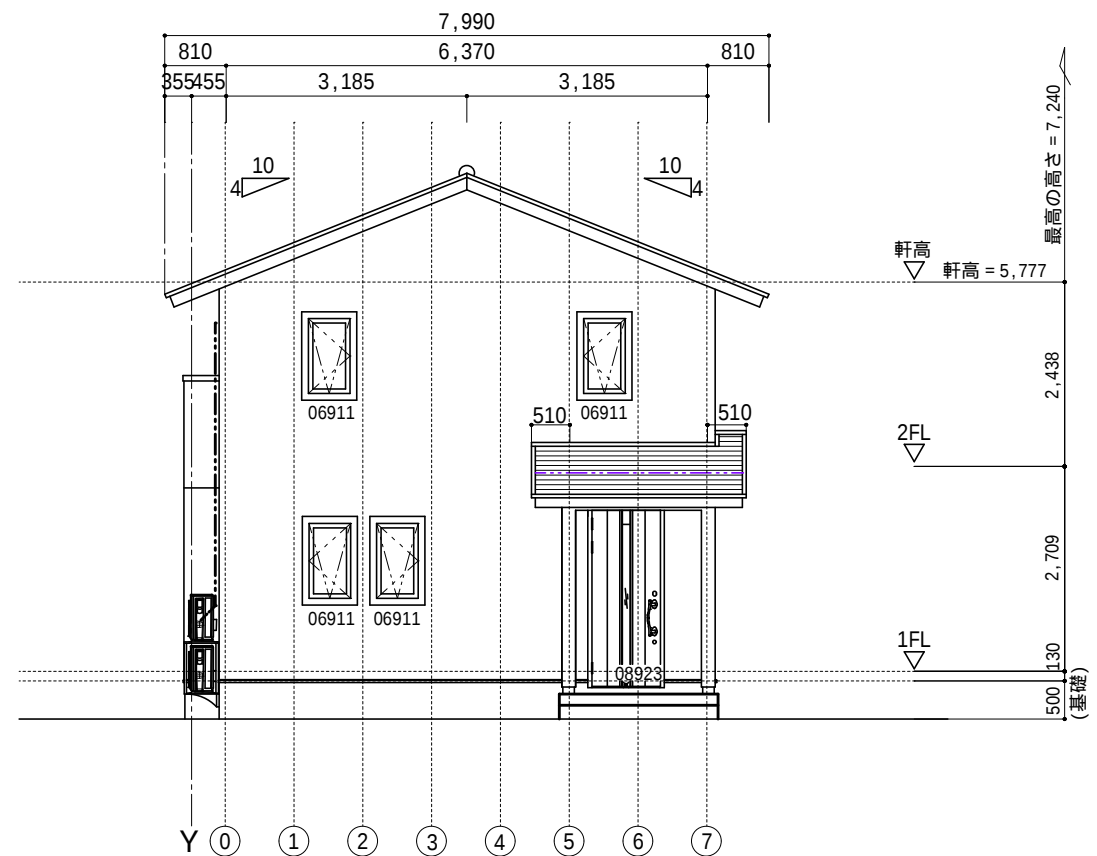
東 立面図
