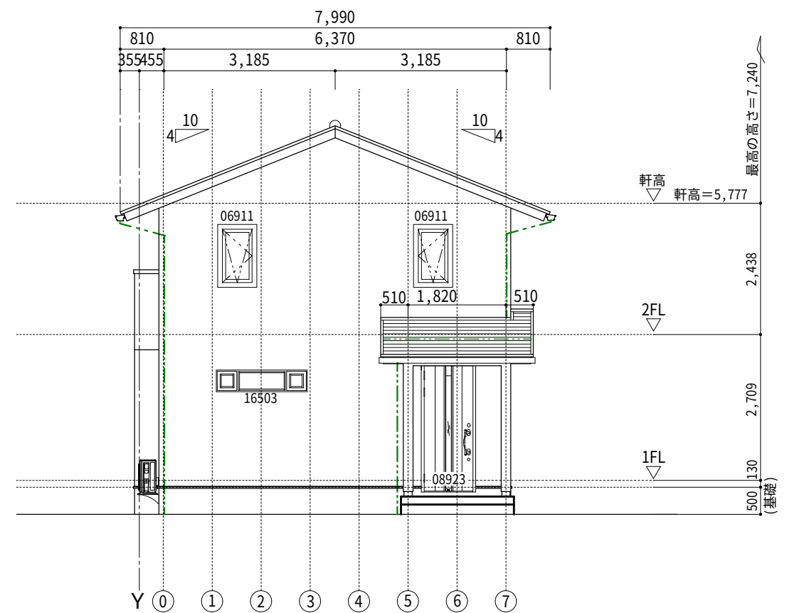
東 立面図
