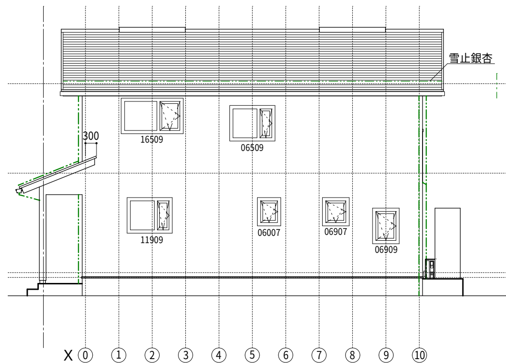
北 立面図
