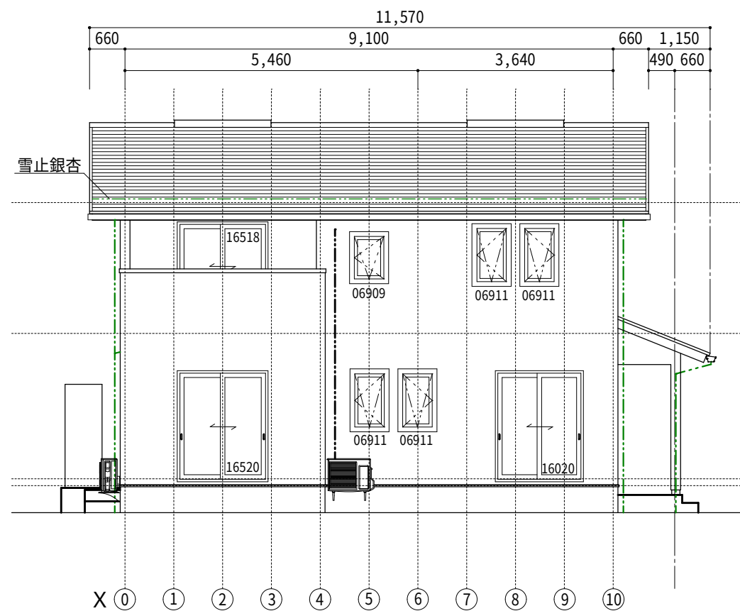
南 立面図
