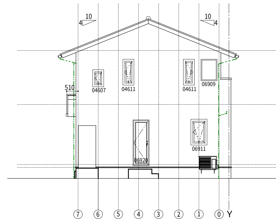
西 立面図
